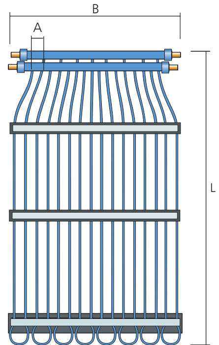
Anschlußvariante 22
