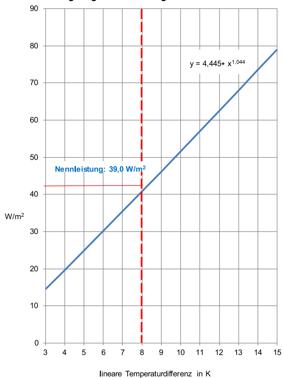
Kühlleistung Singlerohr Baufertigelement B.FR.150
