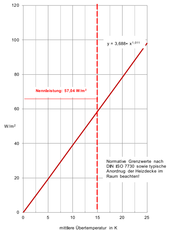
Heizleistung Singlerohr Baufertigelement B.FR.150
